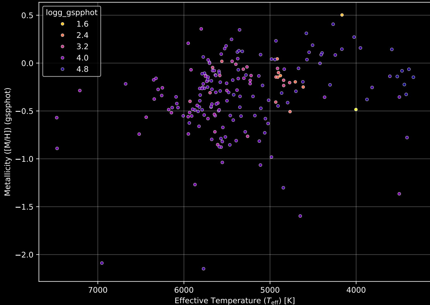
APOGEE DR17 Field: [K2EB_C06_320+48_btx] Stellar Population Parameters (n= 197)
