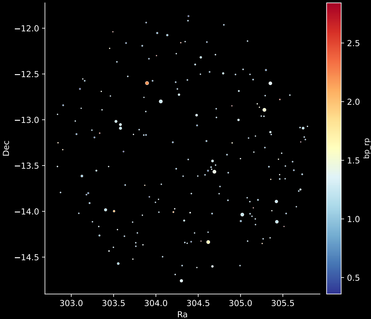
APOGEE DR17 Field: [K2EB_C06_320+48_btx] Stars: 197
